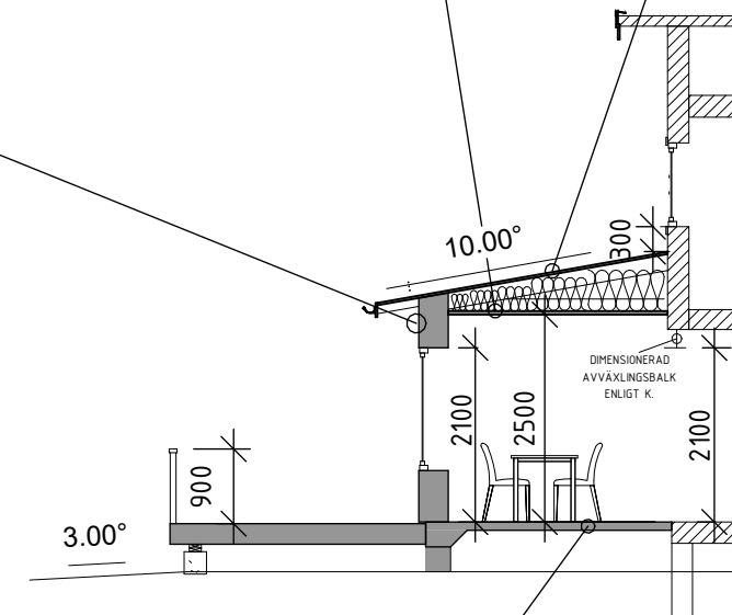
1 SEKTION 1 1 : 100
