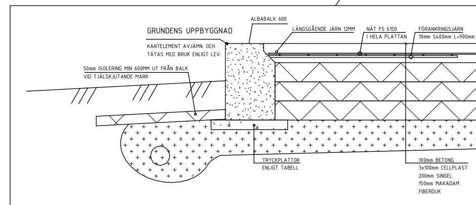
1 SEKTION 1 1 : 100
